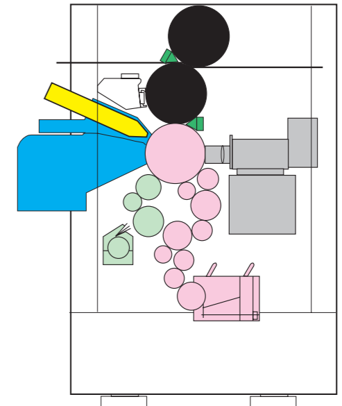
Jednobojana tiskovna jedinica CMY
