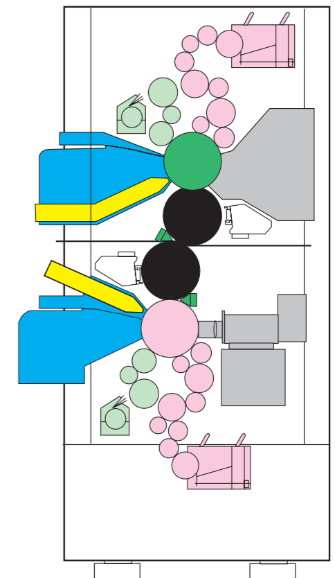
Dvobojana tiskovna jedinica guma-guma (I/I) K
